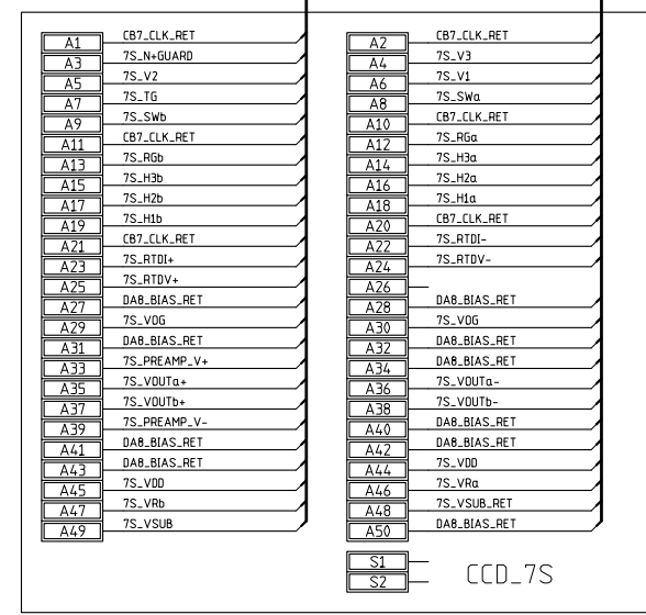
CCD 7S CB 7 DA 8 AMP 104550-6
