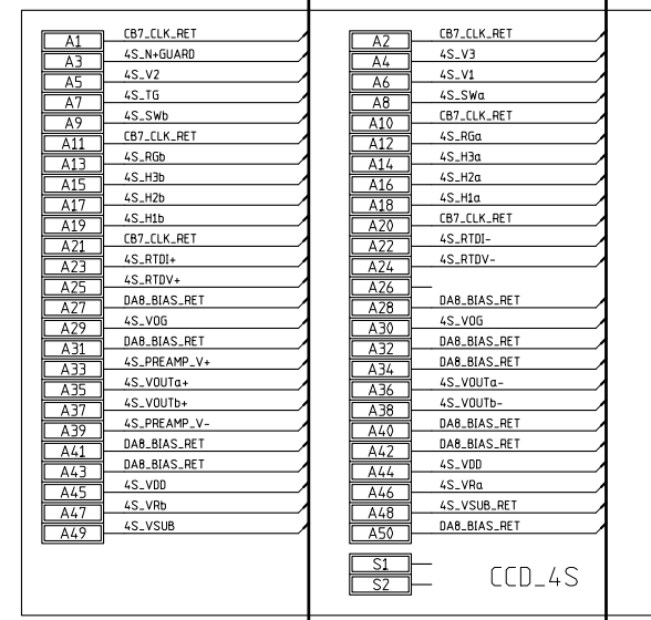
CCD 4S CB 7 DA 8 AMP 104550-6
