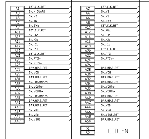
CCD 5N CB 7 DA 9
