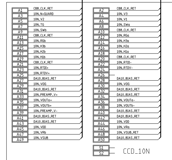
CCD 10N CB 8 DA 10
